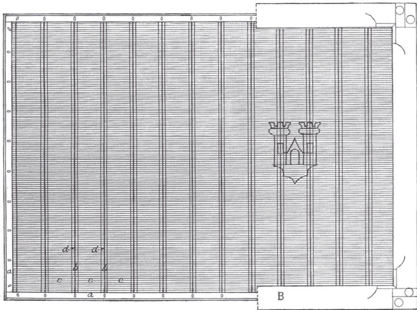
Schematisierte Darstellung eines Schöpfsiebs für die Papierherstellung (nach Piccard)
